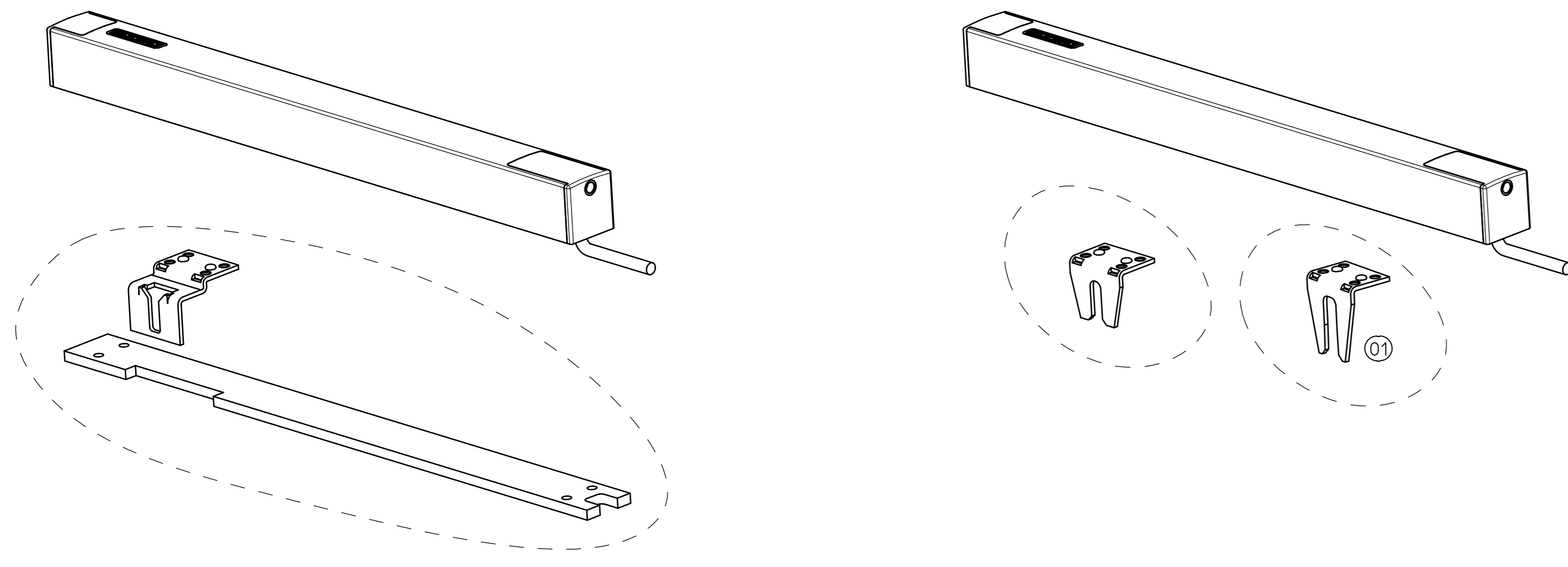
Zubehör Rahmenmontage/ Accessories frame mounting
